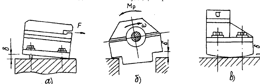
Рис. 4. Снижение жесткости опор:
