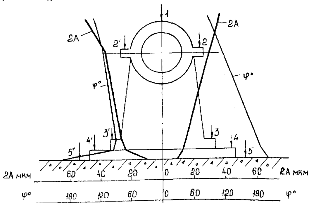
Рис. 3. Контурная характеристика вибрации опоры:
