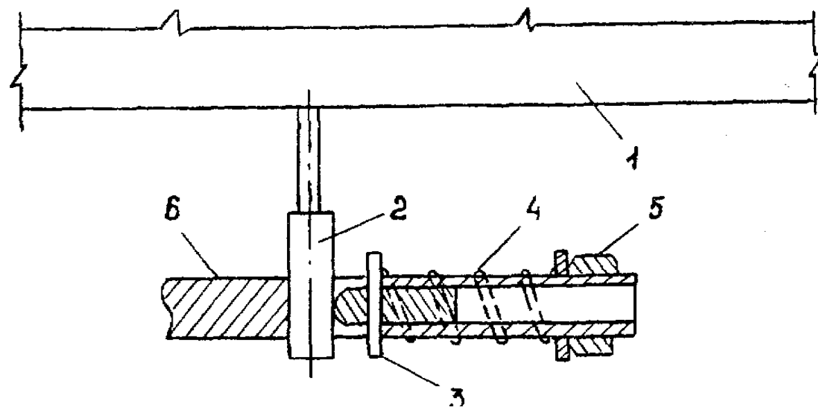
Рис. 8. Демпфер сухого трения:
