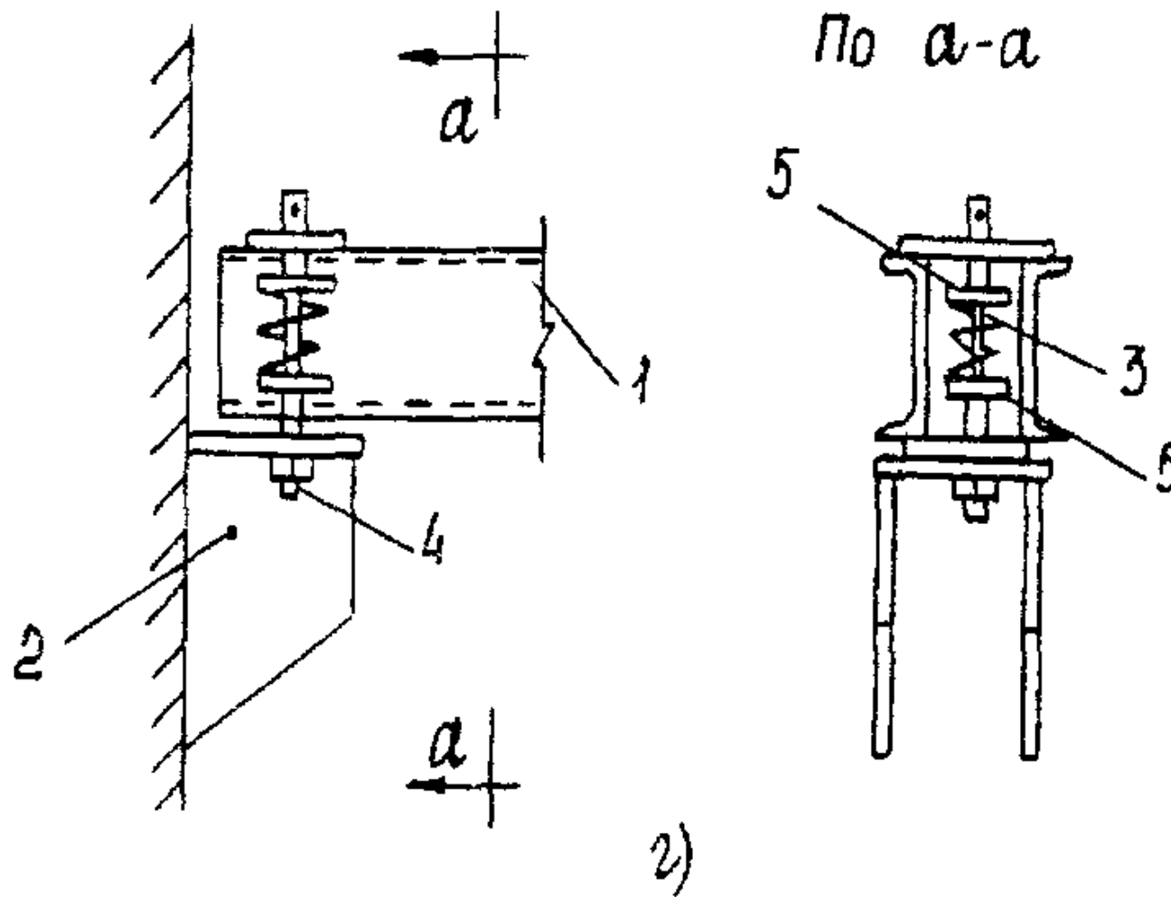
Рис. 6. Отжимно-прижимные приспособления:
