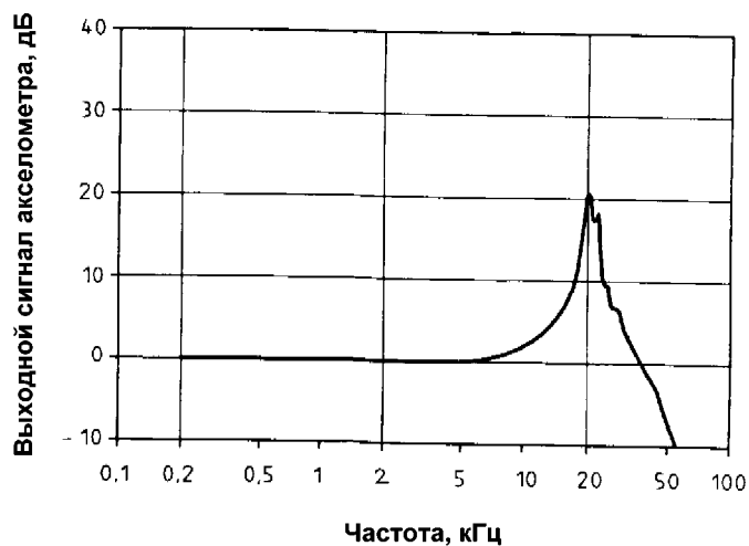
Рисунок 9 — Типичная частотная характеристика акселерометра на магните
