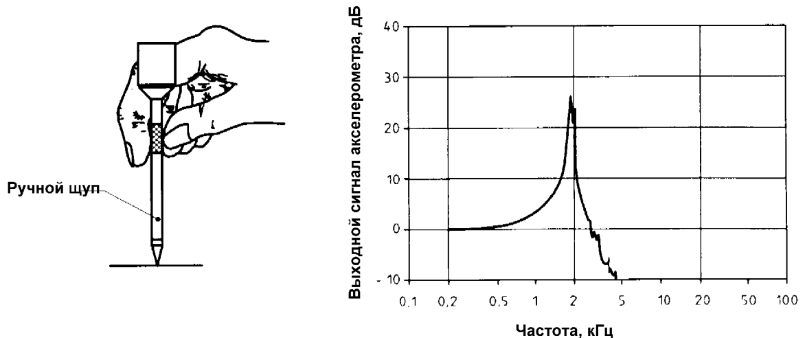
Рисунок 8 — Типичная частотная характеристика акселерометра с щупом
