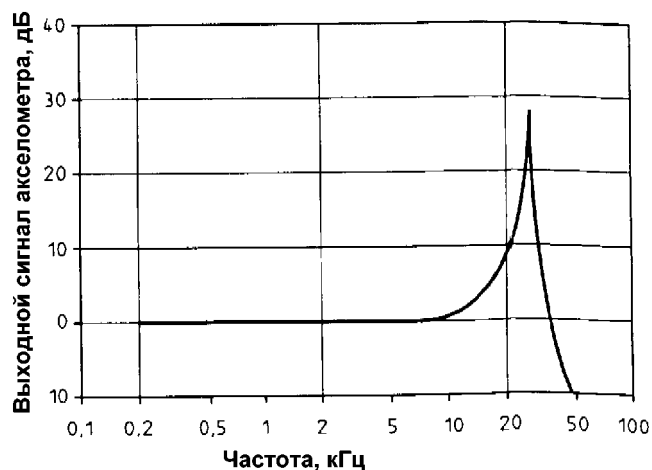
Рисунок 10 — Типичная частотная характеристика акселерометра, установленного на тонкий слой воска
