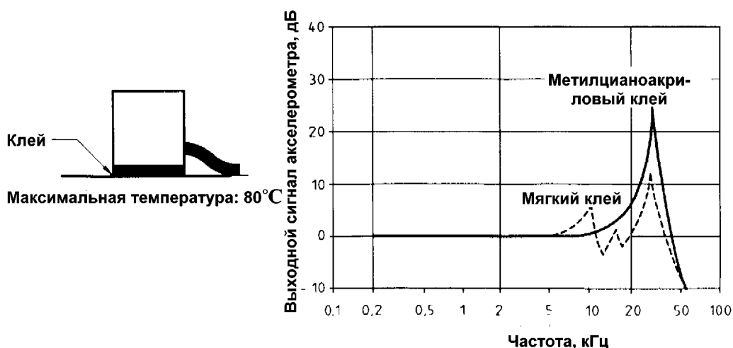
Рисунок 6 — Типичная частотная характеристика акселерометра при клеевом соединении
