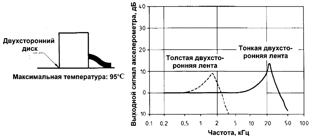
Рисунок 7 — Типичная частотная характеристика акселерометра,
