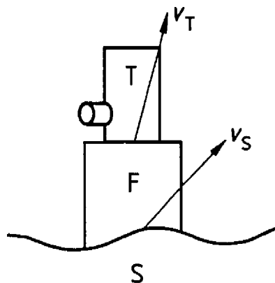
Рисунок 1 — Схематичное изображение установки акселерометра
