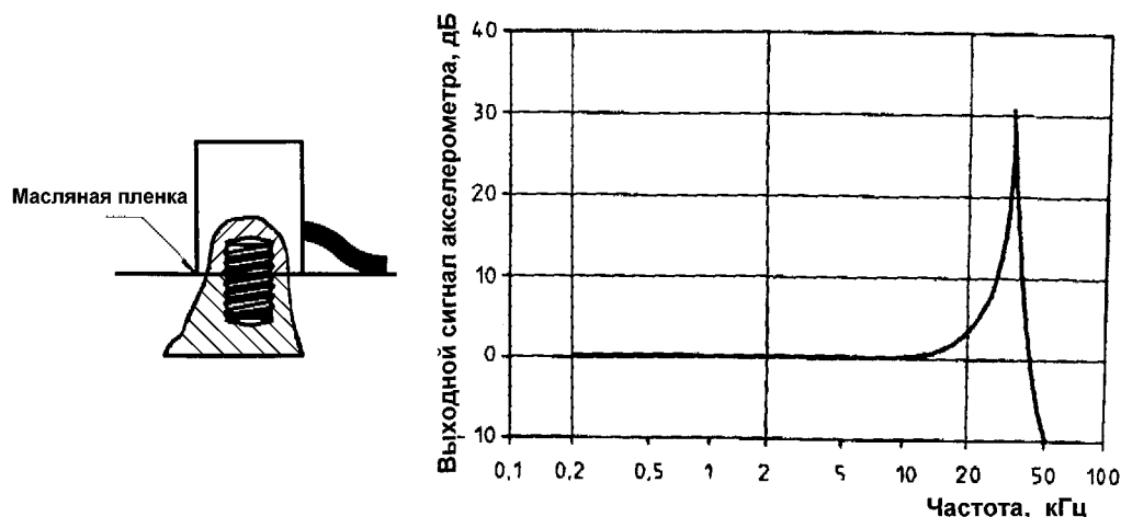
Рисунок 5 — Типичная частотная характеристика акселерометра на шпильке с масляной пленкой в месте крепления
