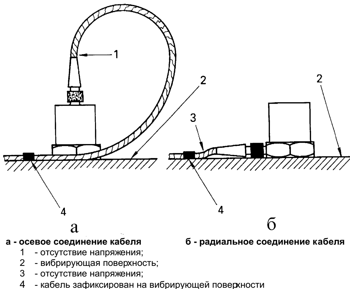
Рисунок 2 — Способы фиксации кабеля для разных типов его соединения с акселерометром
