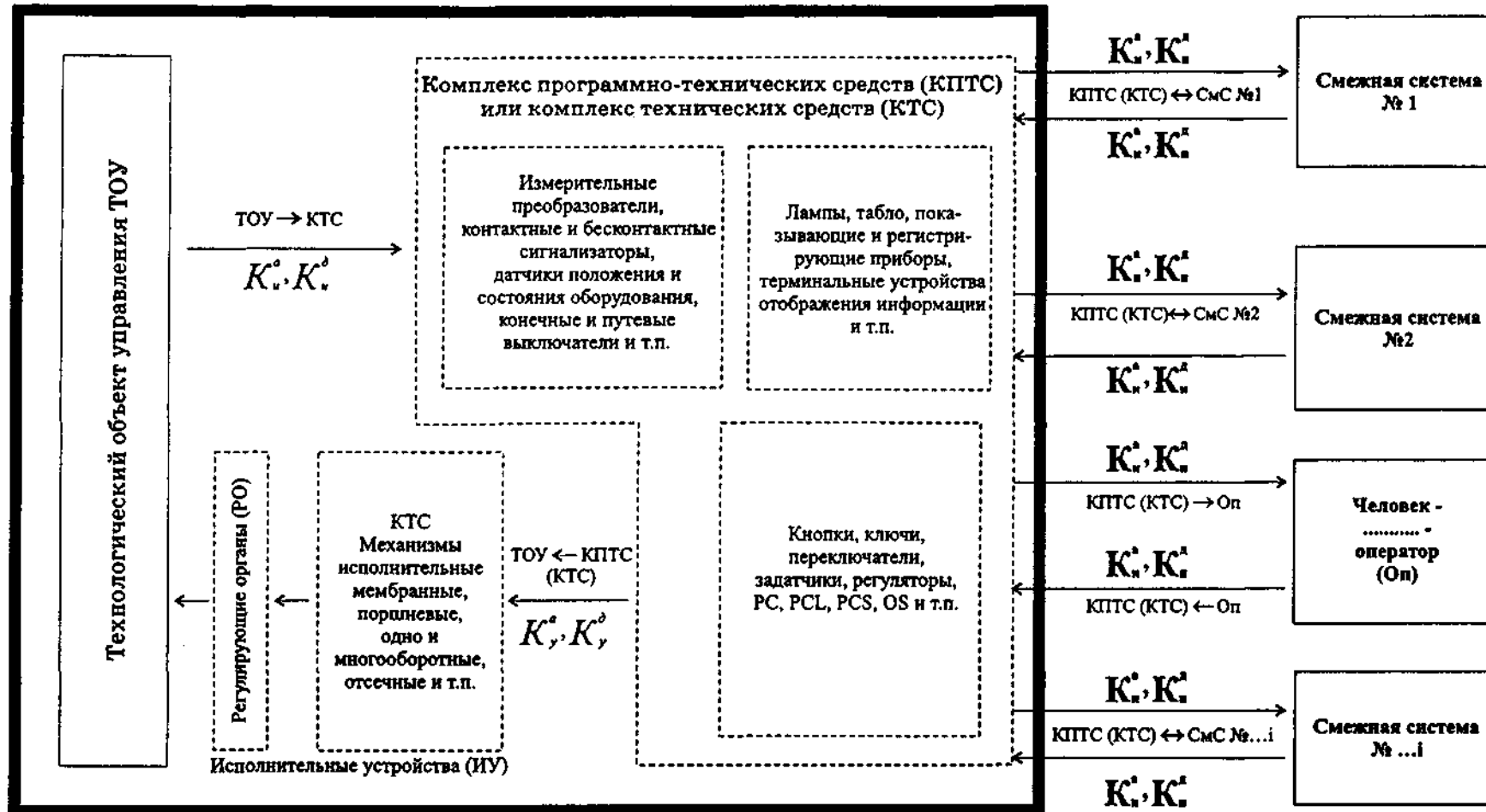
СХЕМА АВТОМАТИЗИРОВАННОГО ТЕХНОЛОГИЧЕСКОГО КОМПЛЕКСА (АТК)
